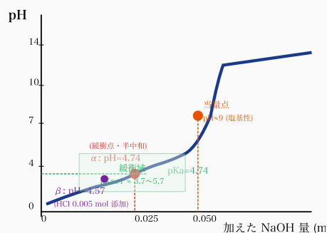
[中和滴定曲線 — 酢酸 NaOH 滴定]
