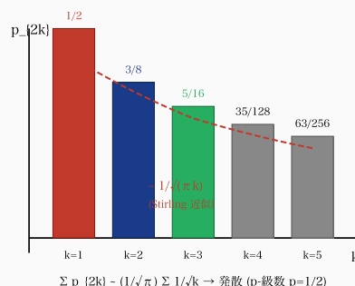
[原点復帰確率 p_{2k} の減衰 (Stirling 近似)]
