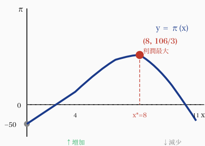
利潤関数 \pi(x) = -(1/3)x^3 + 4x^2 - 50 のグラフ
