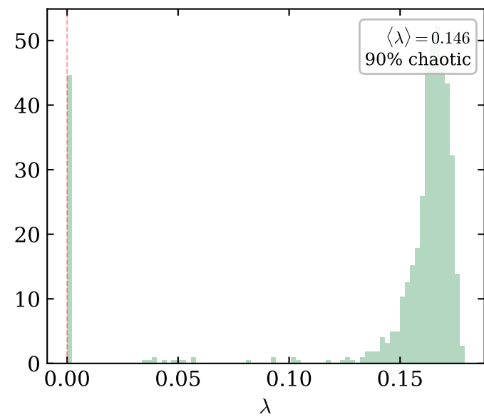
(d) Stadium FTLE, \alpha = 1.0
