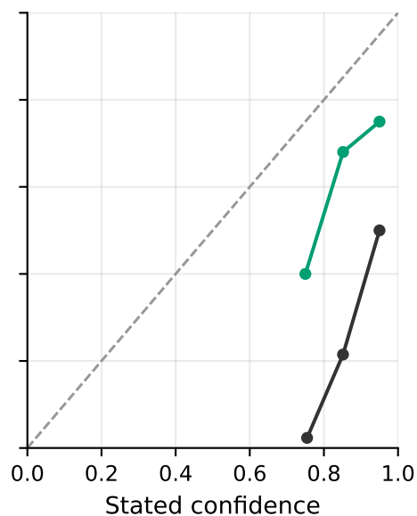
Gemma4-E2B
