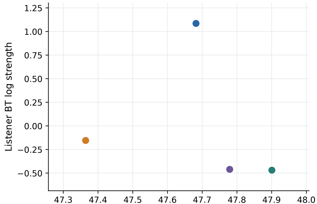
HSC-MSC
