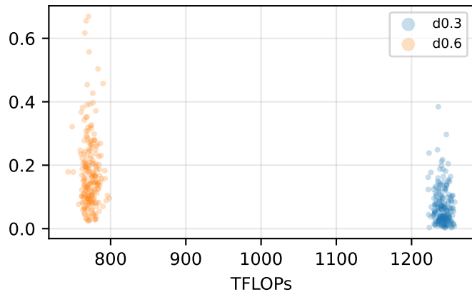
Wan LPIPS per prompt
