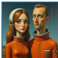
ReSPect (ours)
