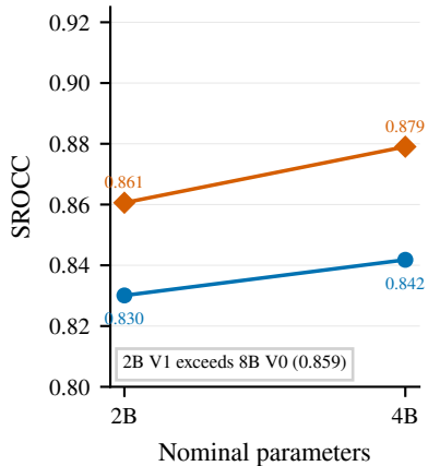
(c) Qwen3-VL
