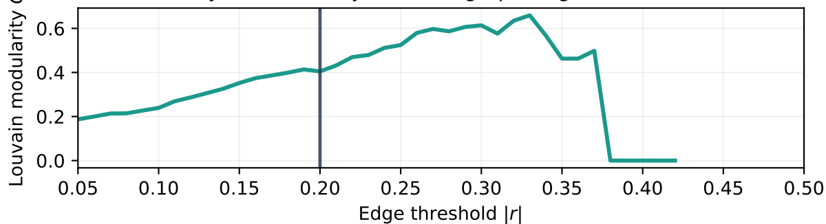
(d) Modularity (rises trivially once the graph fragments)
