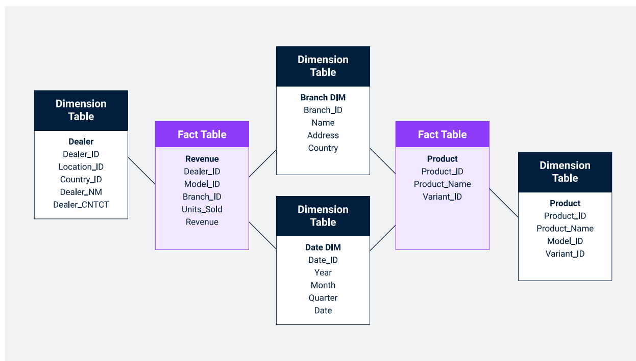
Dig 3 : Galaxy Schema
