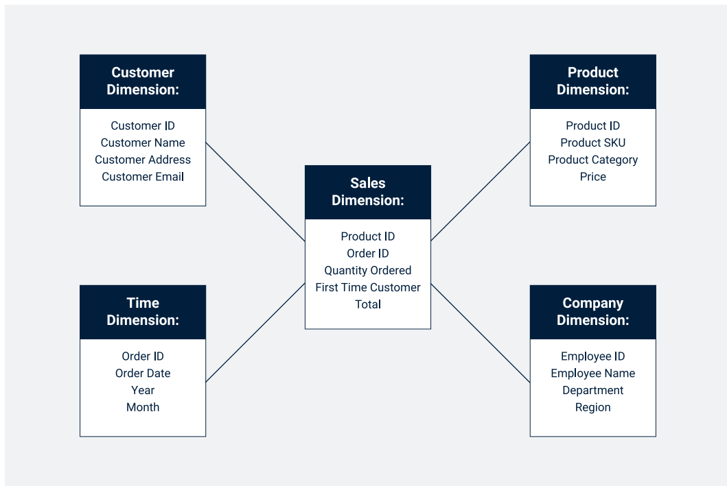
Dig 1 : Star Schema
