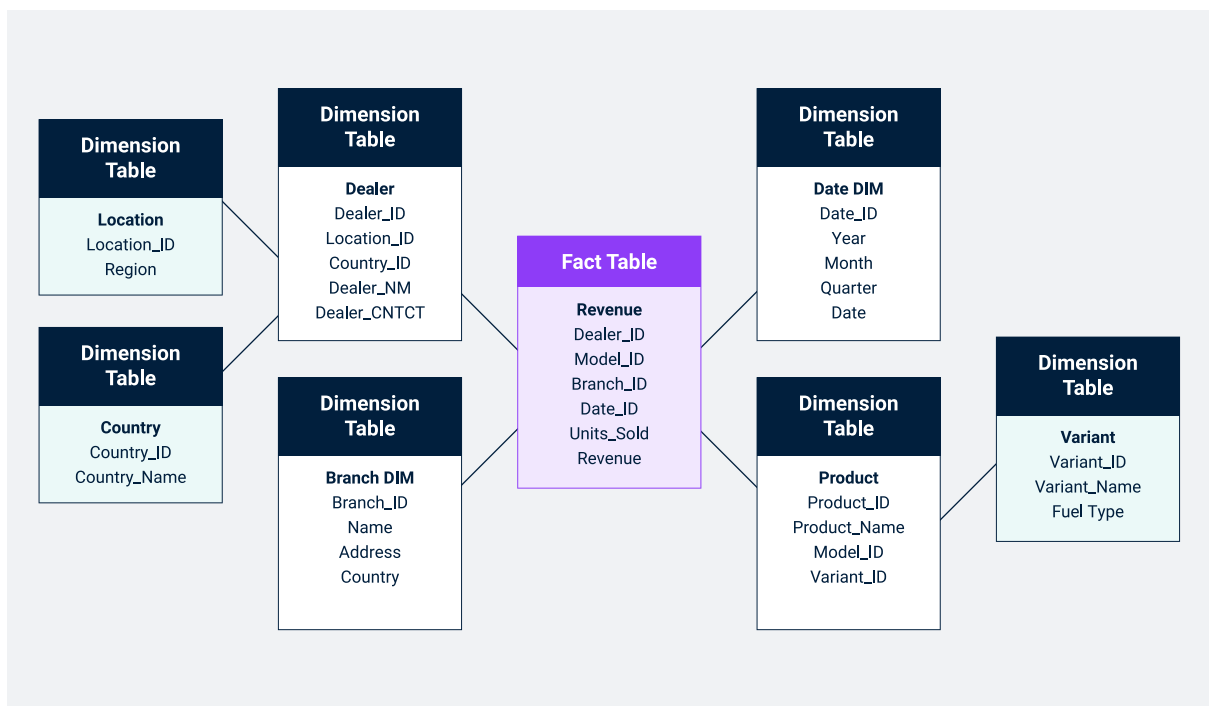
Dig 2 : Snowflake Schema
