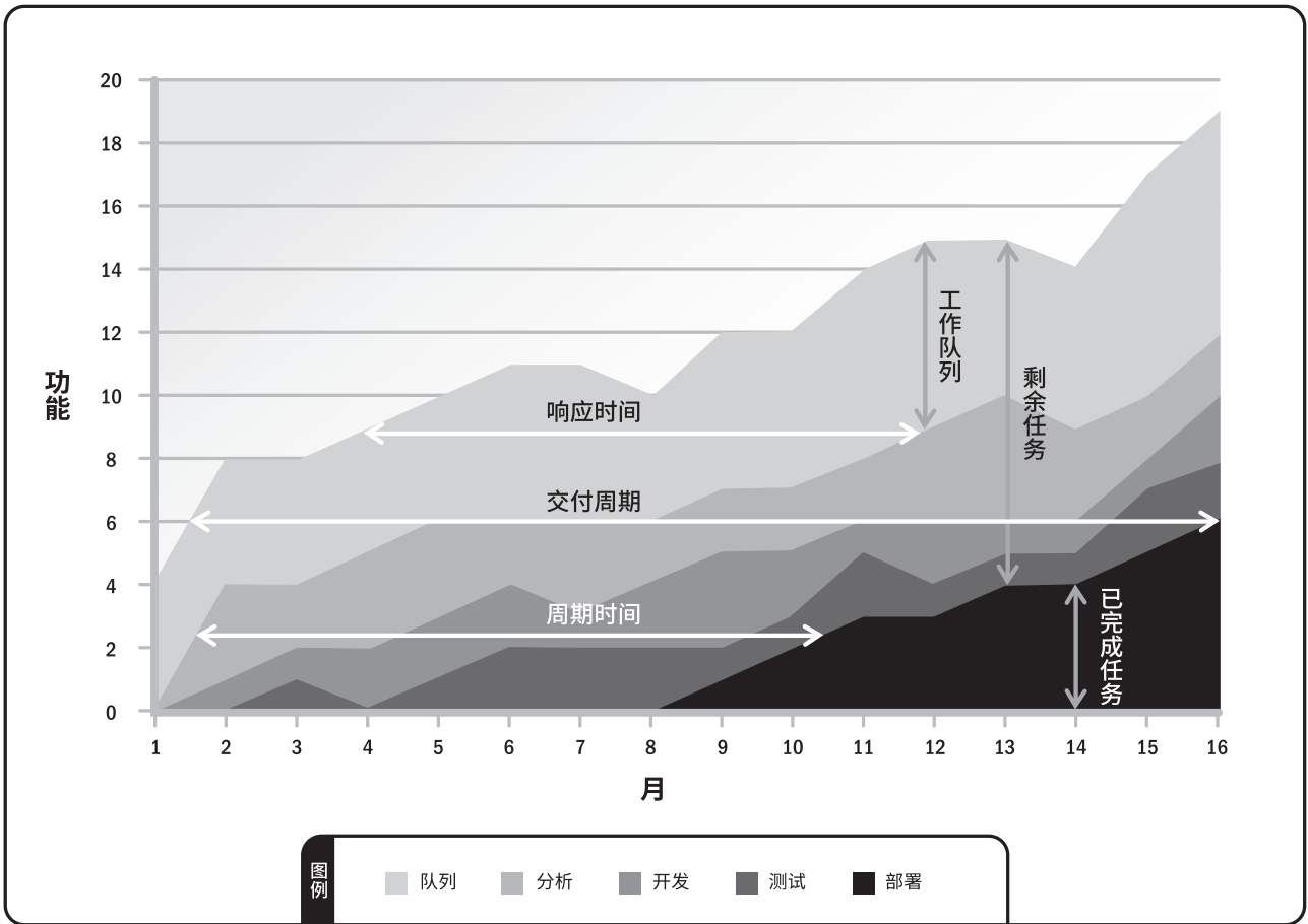
图 5-7 已完成功能的累积流图
