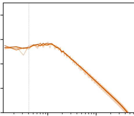
hel2 (helical)
