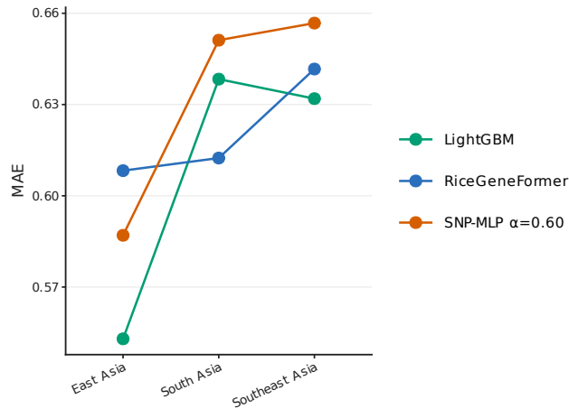
d Ordinal MAE under region shift
