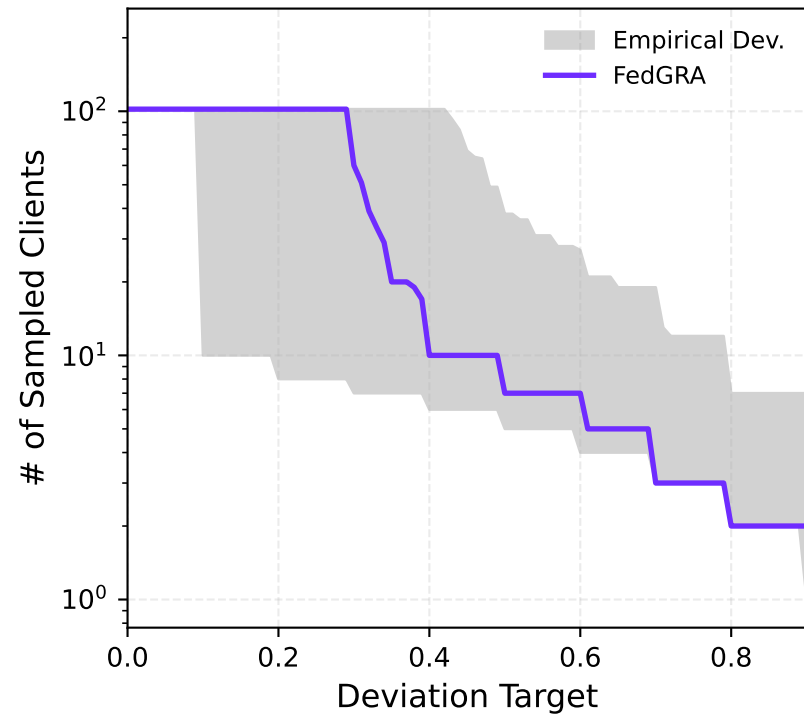
FedGRA
