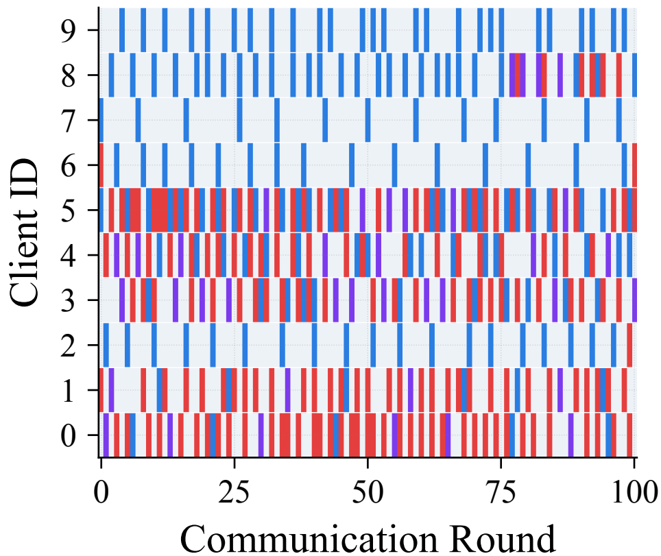
MNIST
