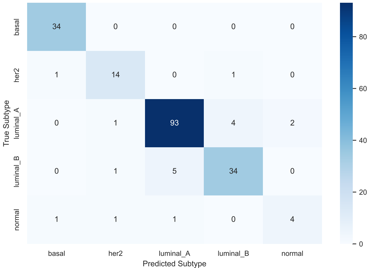
Confusion Matrix: MLP
