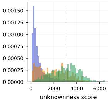
Mahalanobis
