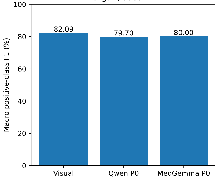
Organ; seed 42
