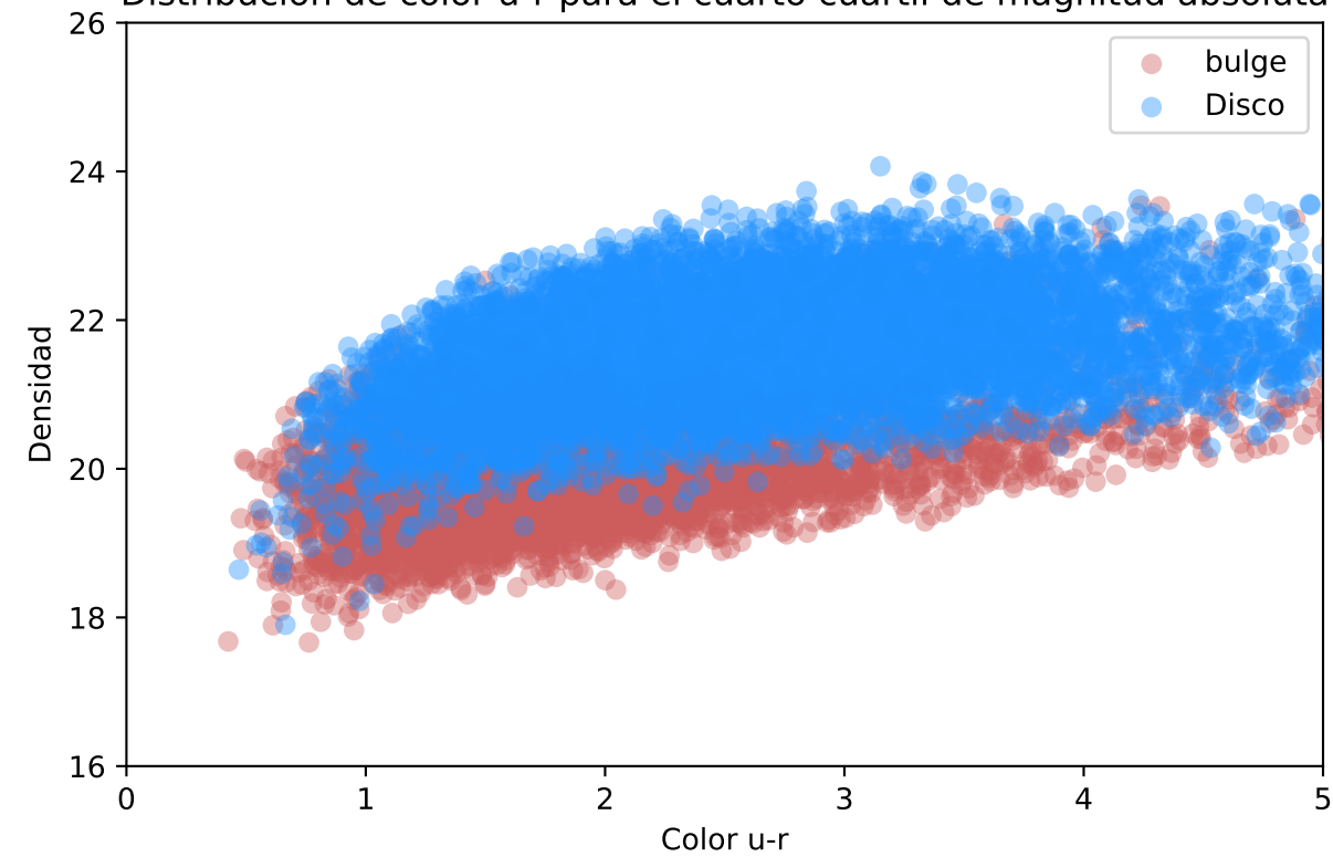
Distribución de color u-r para el cuarto cuartil de magnitud absoluta
