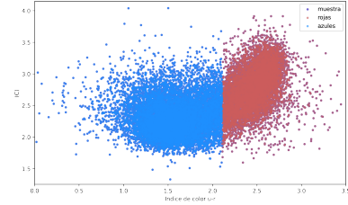
Figura 10: Diagrama comparación parámetro de concentración vs índice de color de u - r
