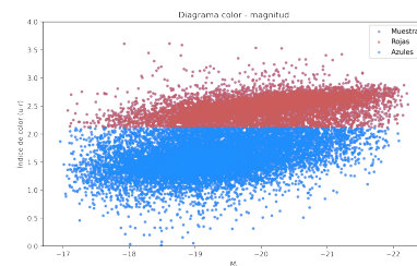
Figura 15: Diagrama color magnitud para galaxias rojas y azules.
