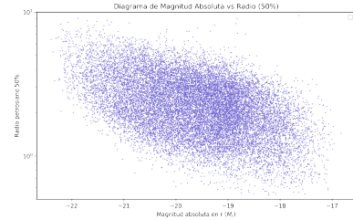
Figura 11: Diagrama tamaño vs luminosidad para toda la muestra de galaxias.
