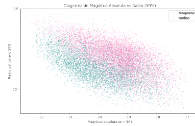
Figura 14: Diagrama tamaño vs luminosidad para galaxias tempranas en color o tardías en color
