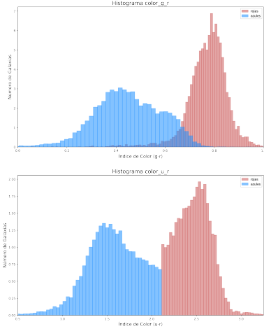
Figura 6: Histograma de los índices de color de las galaxias rojas y azules.
