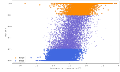
Figura 9: Diagrama comparación parámetro de concentración vs parametro de fracDeV
