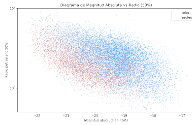
Figura 12: Diagrama tamaño vs luminosidad para galaxias rojas y azules.
