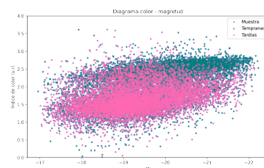
Figura 17: Diagrama color magnitud para galaxias tempranas en color o tardías en color
