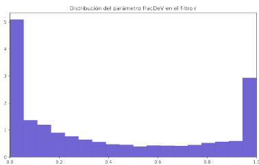
Figura 8: Histograma del parametro de fracDeV
