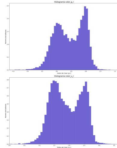
Figura 5: Histograma de los índices de color de las galaxias seleccionadas.
