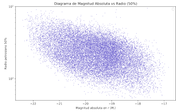
Figure 11: Diagrama tamaño vs luminosidad para toda la muestra de galaxias.
