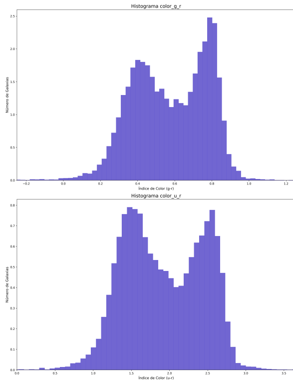
Figure 5: Histograma de los índices de color de las galaxias seleccionadas.
