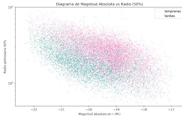
Figure 14: Diagrama tamaño vs luminosidad para galaxias tempranas en color o tardías en color
