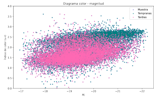
Figure 17: Diagrama color magnitud para galaxias tempranas en color o tardías en color
