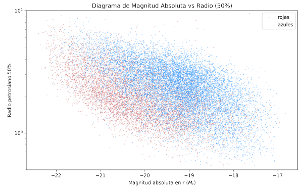
Figure 12: Diagrama tamaño vs luminosidad para galaxias rojas y azules.
