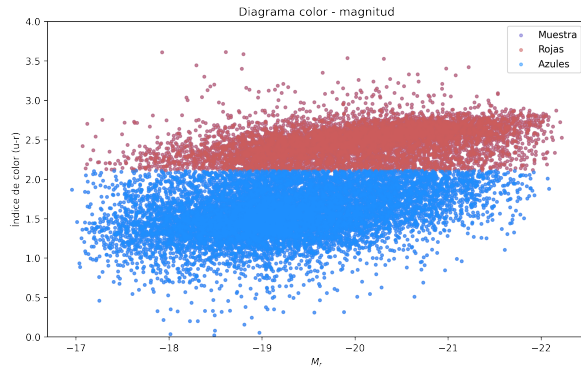
Figure 15: Diagrama color magnitud para galaxias rojas y azules.
