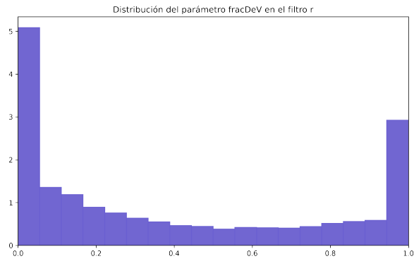
Figure 8: Histograma del parámetro de fracDeV
