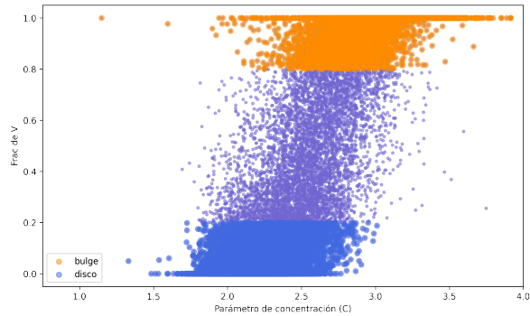
Figure 9: Diagrama comparación parámetro de concentración vs parámetro de fracDeV
