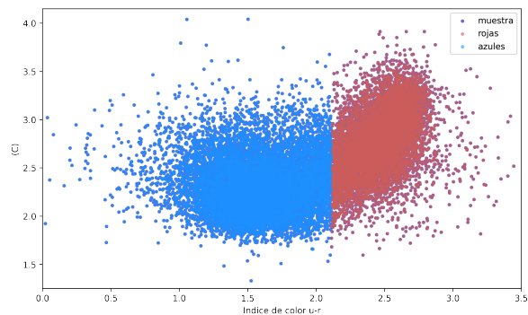
Figure 10: Diagrama comparación parámetro de concentración vs índice de color de u - r
