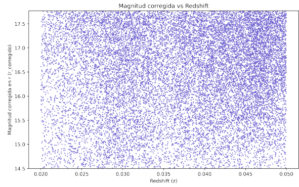
Magnitud aparente en la banda r corregida por extinción, como función del redshift.
