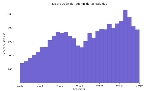
Distribución del redshift de las galaxias de la muestra.
