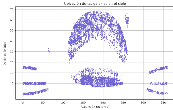
Distribución de las galaxias de la muestra en el diagrama de coordenadas (alfa,delta)
