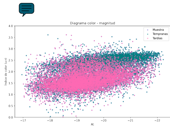
Figure 18: Diagrama color magnitud para galaxias tempranas en color o tardías en color
