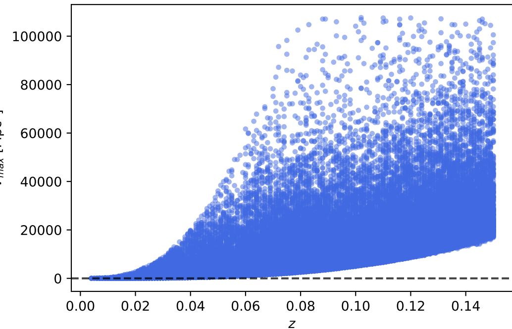
Volumen máximo de galaxias en función del corrimiento al rojo
