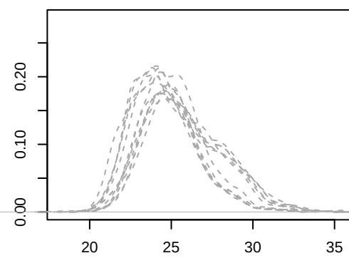
CycLoess
