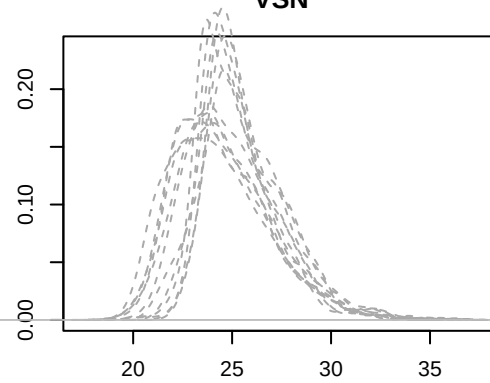
VSN
