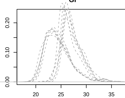
GI
