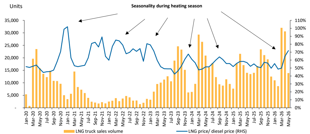
Figure 17 - LNG truck sales volume vs. LNG/diesel price
