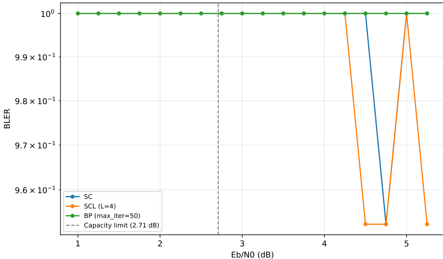
SC vs SCL vs BP (N=256)
