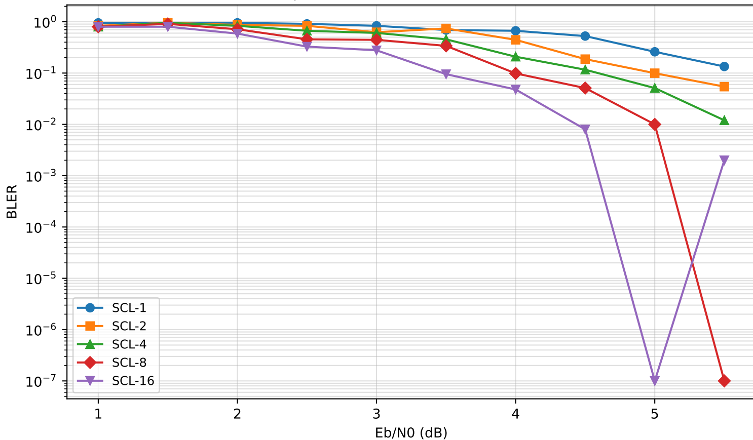
Exp2: SCL list size (N=128, K=64)
