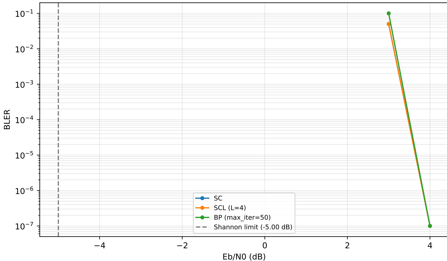
SC/SCL/BP N=256
