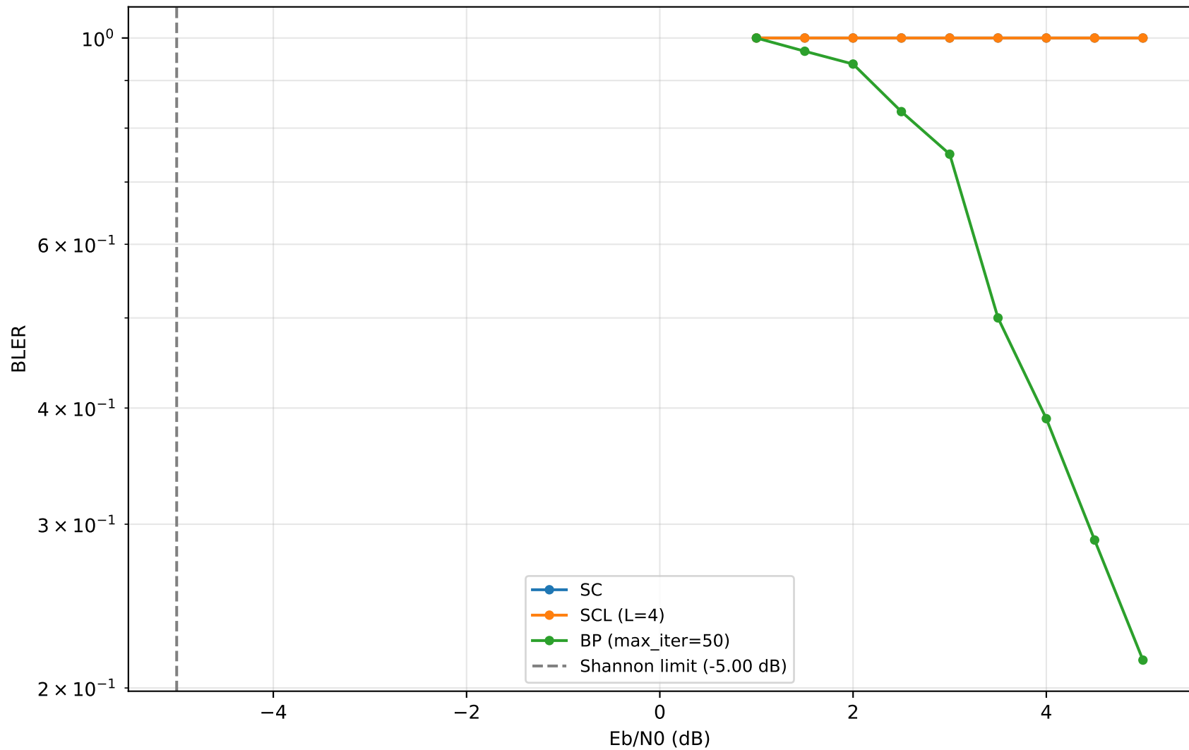
SC vs SCL vs BP (N=256)
