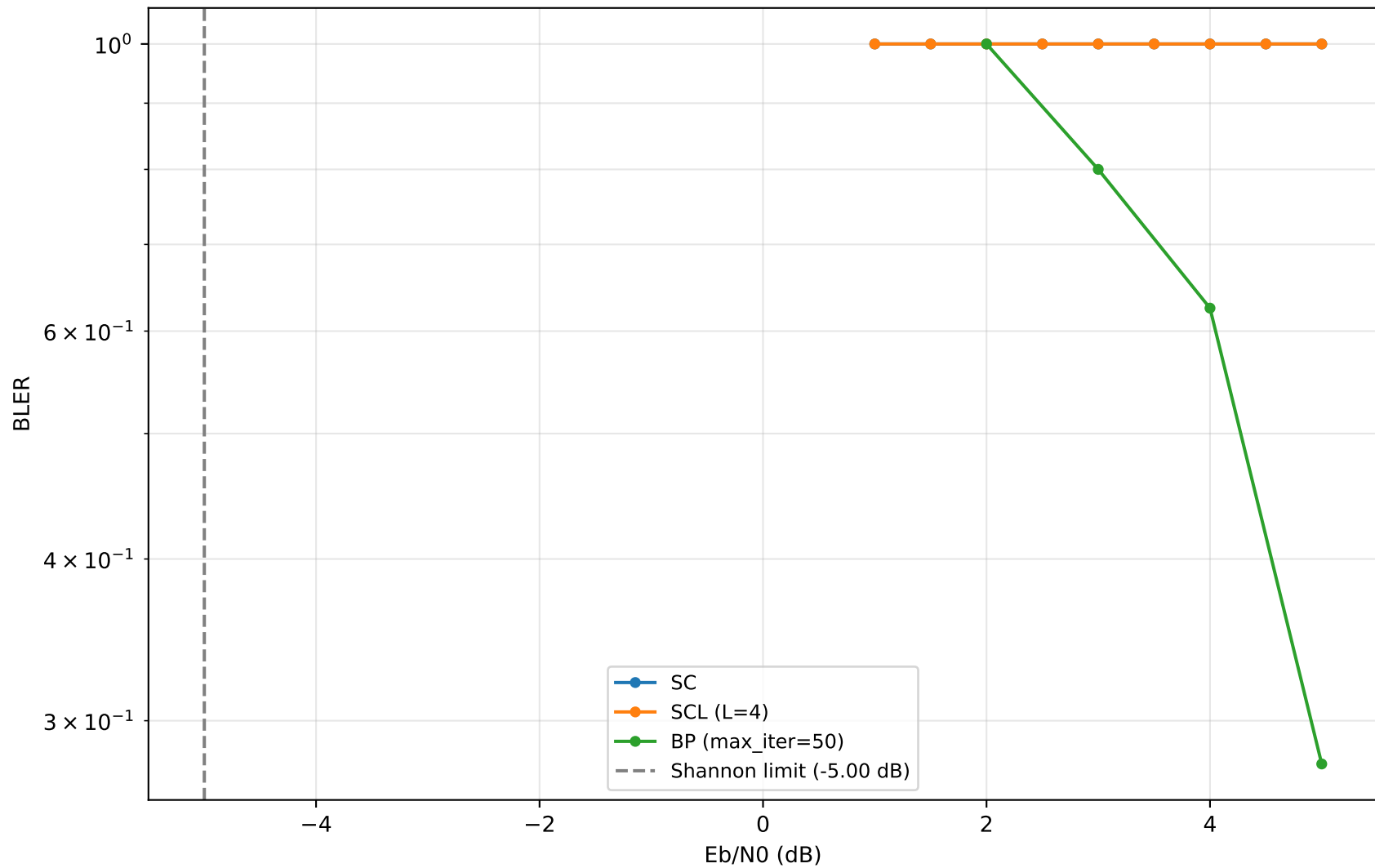
SC vs SCL vs BP (N=512)
