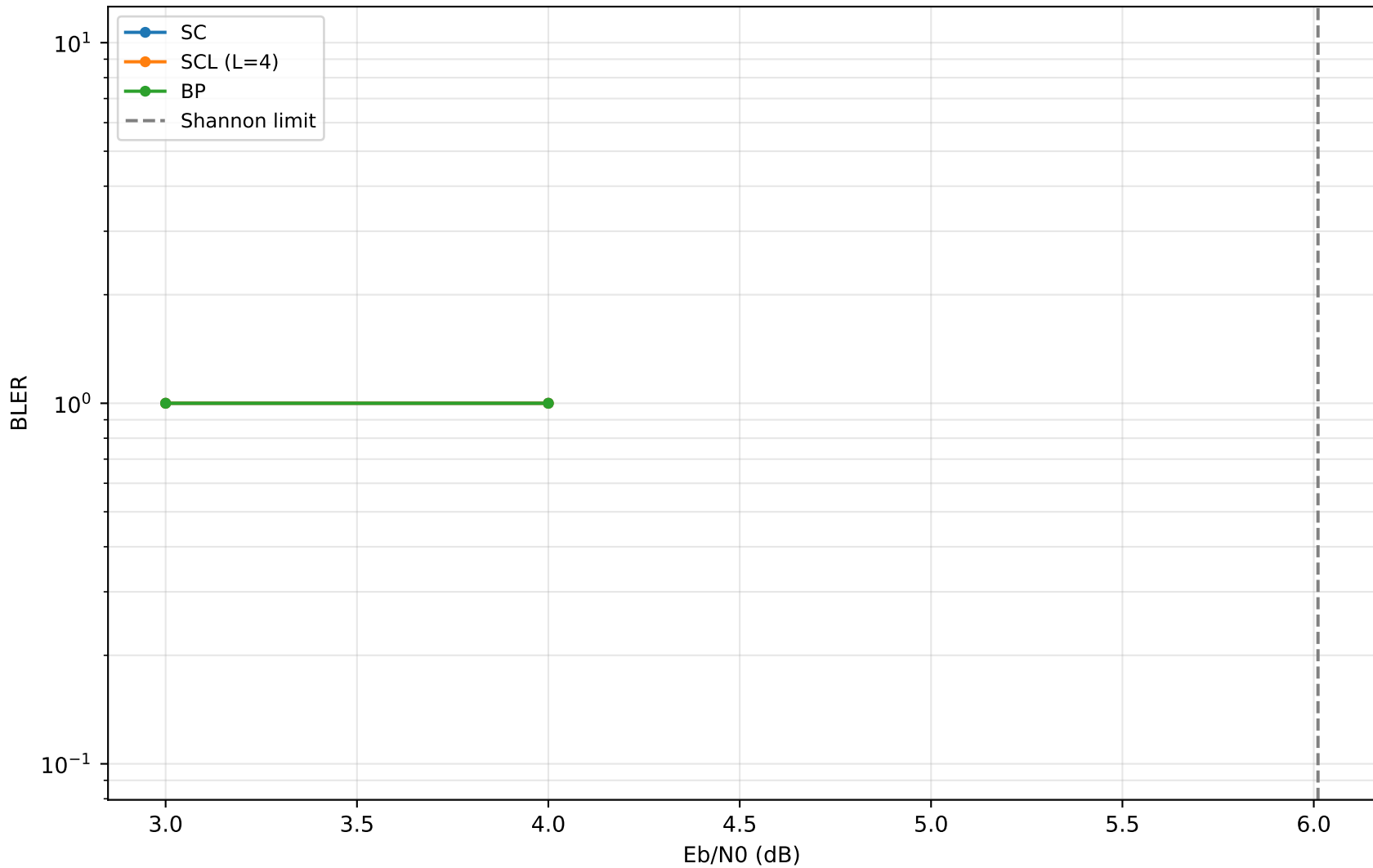
SC vs SCL vs BP N=256
