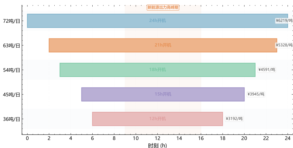
图 5-9: 各产量水平最优开机时段安排
