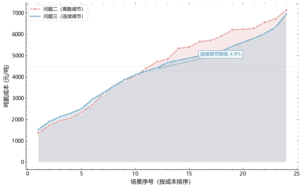
图 6-15: 全年吨氨成本分布曲线（问题二与问题三对比）
