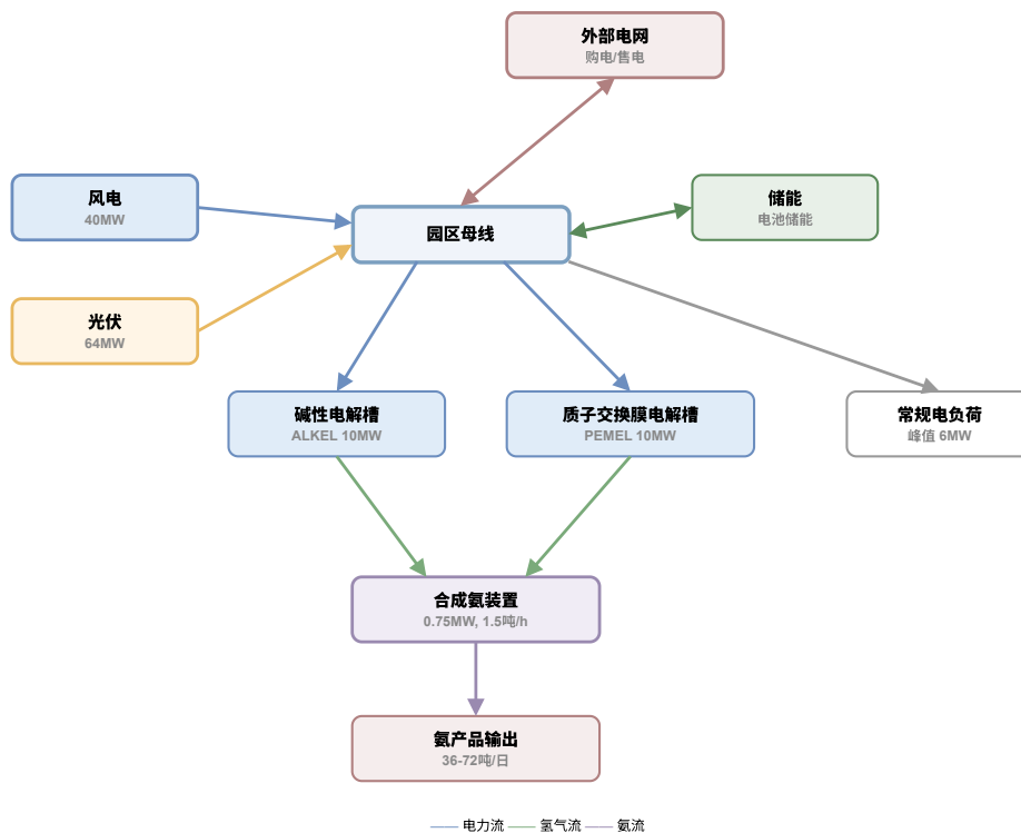
图 1-2: 绿电直连型电氢氨园区能量流拓扑图
