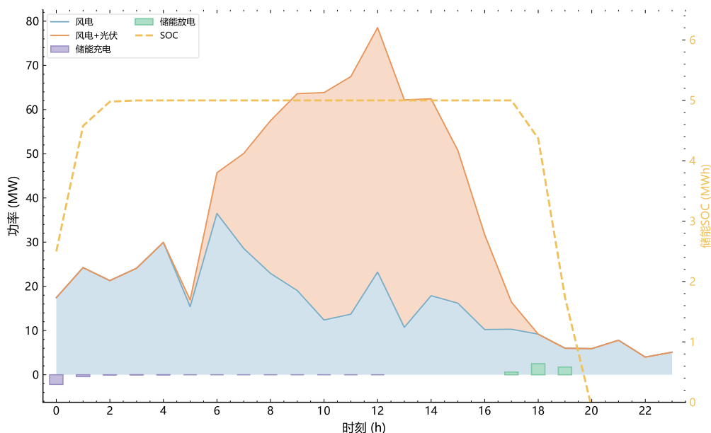
图 7-18: 最大弃电场景储能充放电调度方案
