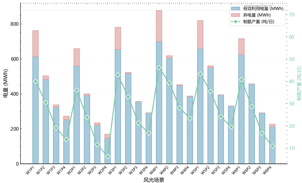
图 7-17: 24 场景离网产量与电量利用分布
