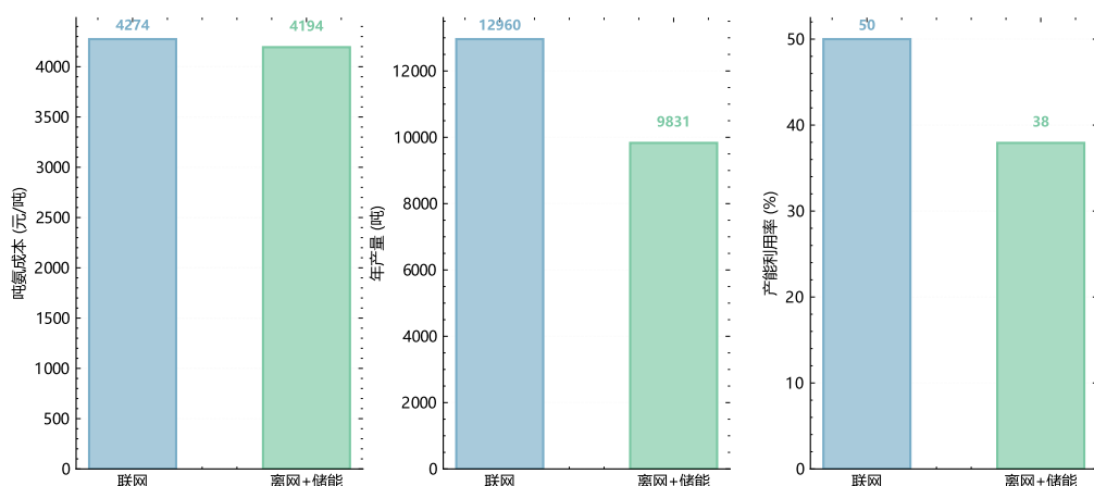
图 7-19: 离网与联网运行模式经济性对比
