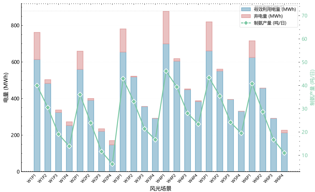
图 7-17: 24 场景离网产量与电量利用分布
