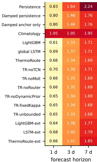
(a) Pooled RMSE (°C)
