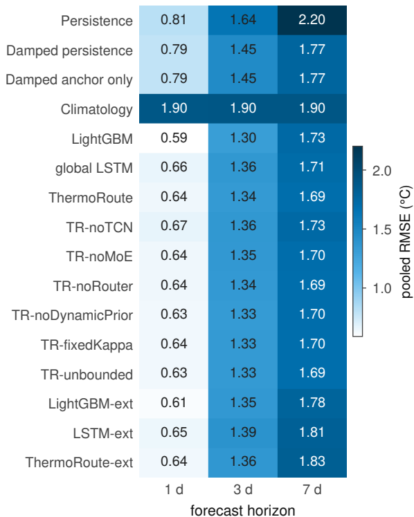
(a) Pooled RMSE (°C)
