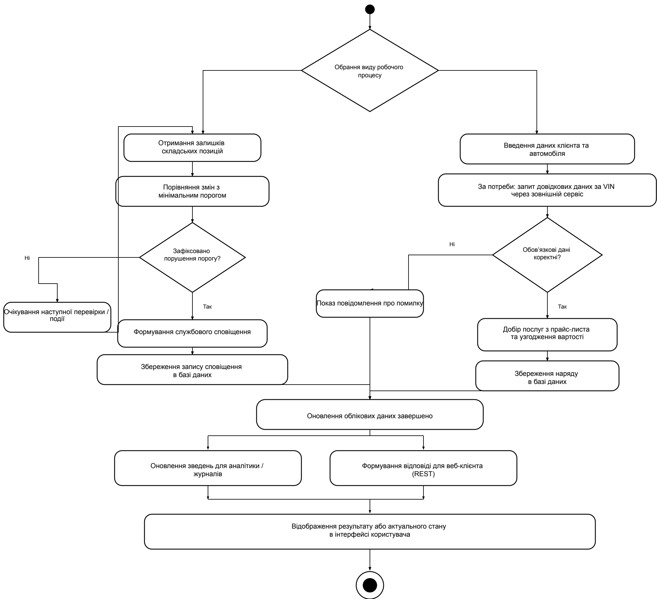
Діаграма діяльності STO CRM
