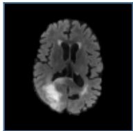
FLAIR
