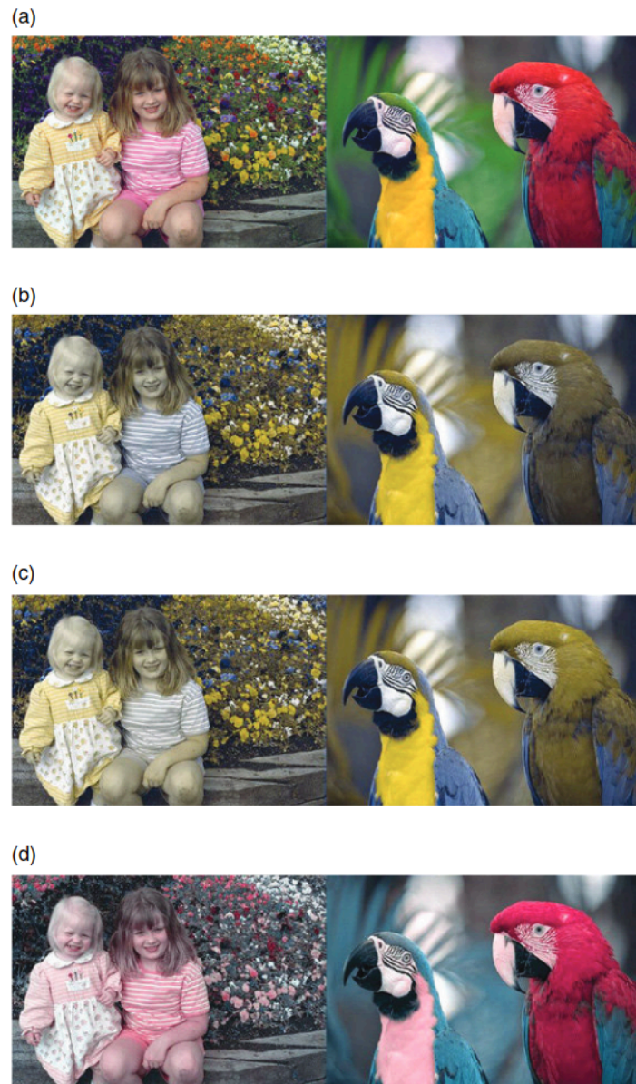
图 1.22：展示各种色觉缺陷患者的色彩辨别能力：(a) 原始图像，(b) 红色盲，(c) 绿色盲，(d) 蓝色盲。
