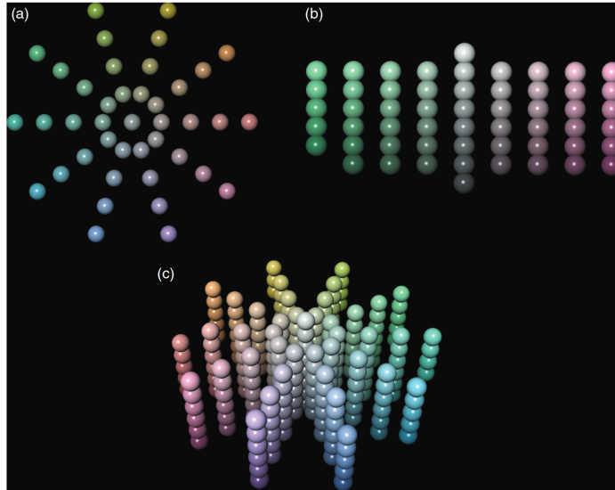
图5.3：孟塞尔系统样本的颜色渲染图 (a) 定明度平面，(b) 一对定色相平面，(c) 三维透视图
