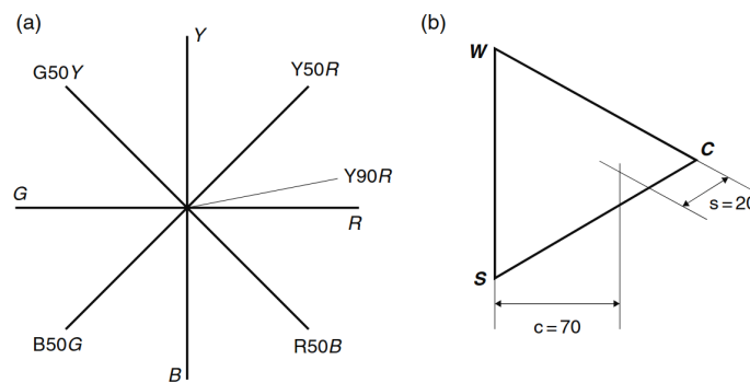
图5.5: (a) NCS系统的色相圆和(b) 常色相黑度/色度平面的图示
