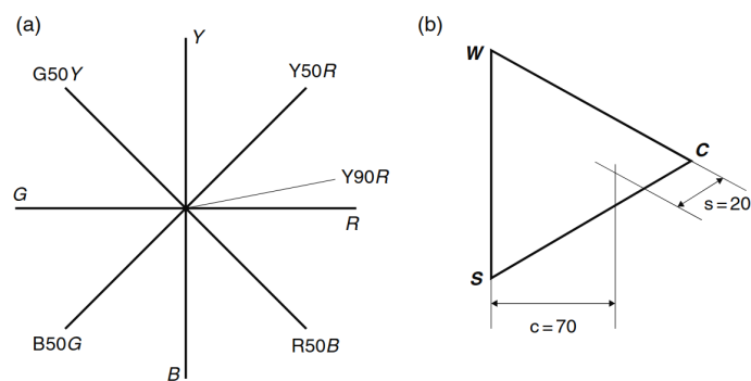
图5.5：Colorcurve系统的图示，展示了色相圆和常色相黑度/色度平面的图示
