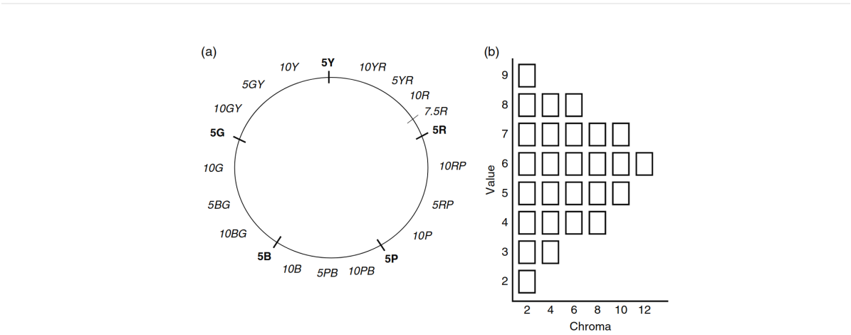
图5.2：图示（a）孟塞尔色相圆和（b）定色相的明度/色度平面
