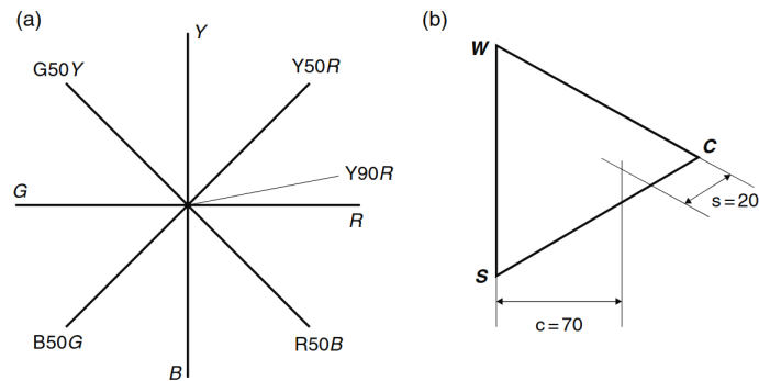
图5.5：Colorcurve系统的图示，展示了色调圆和常色调黑度/色度平面的图示
