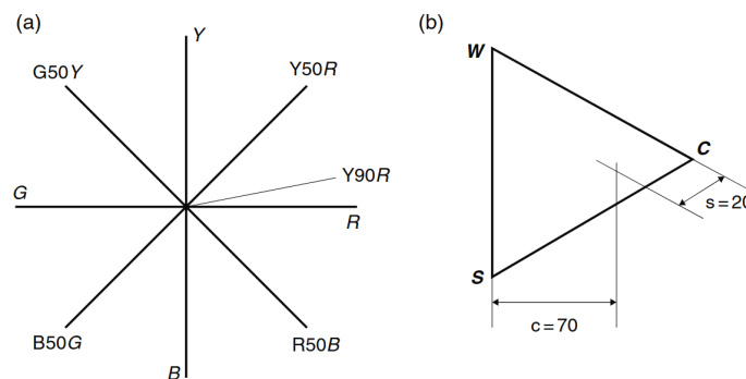
图5.5: (a) NCS系统的色调圆和(b) 常色调黑度/色度平面的图示
