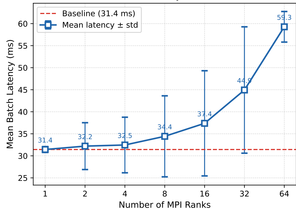
(d) Per-Batch Latency vs. MPI Ranks
