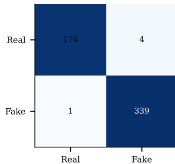
(c) FSTT-Net confusion
