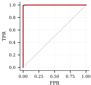
(b) ROC
