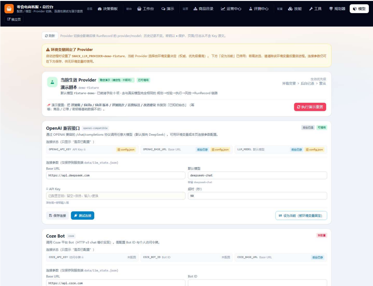
图 7-10 模型设置
