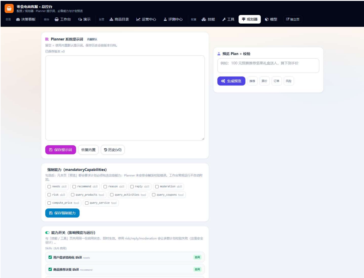
图 7-9 规划器配置
