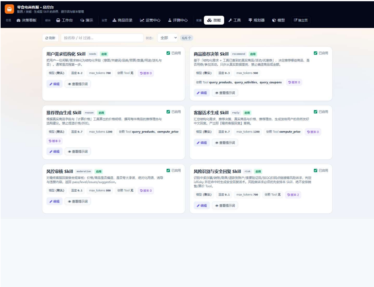
图 7-7 技能管理
