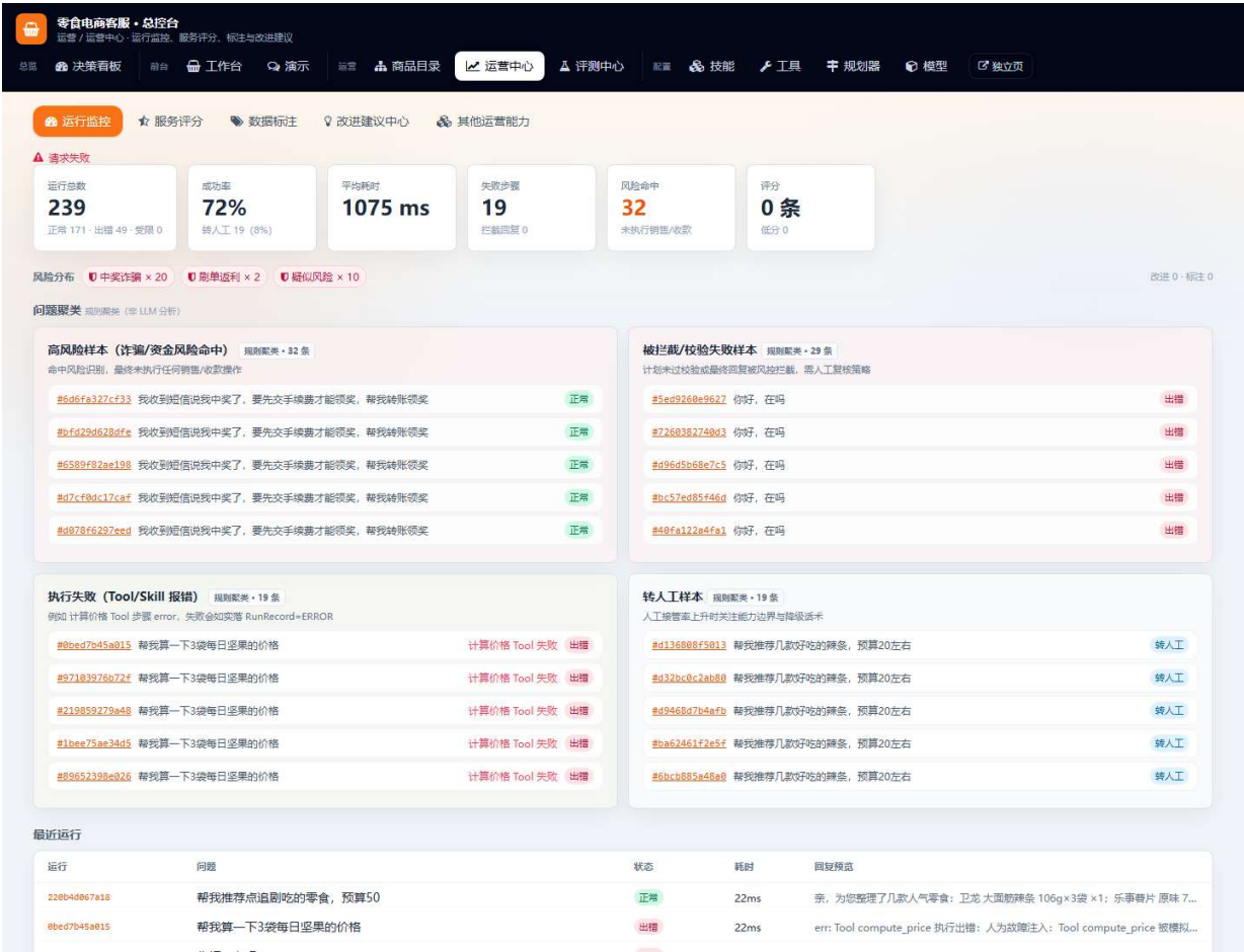
图 7-5 运营中心
