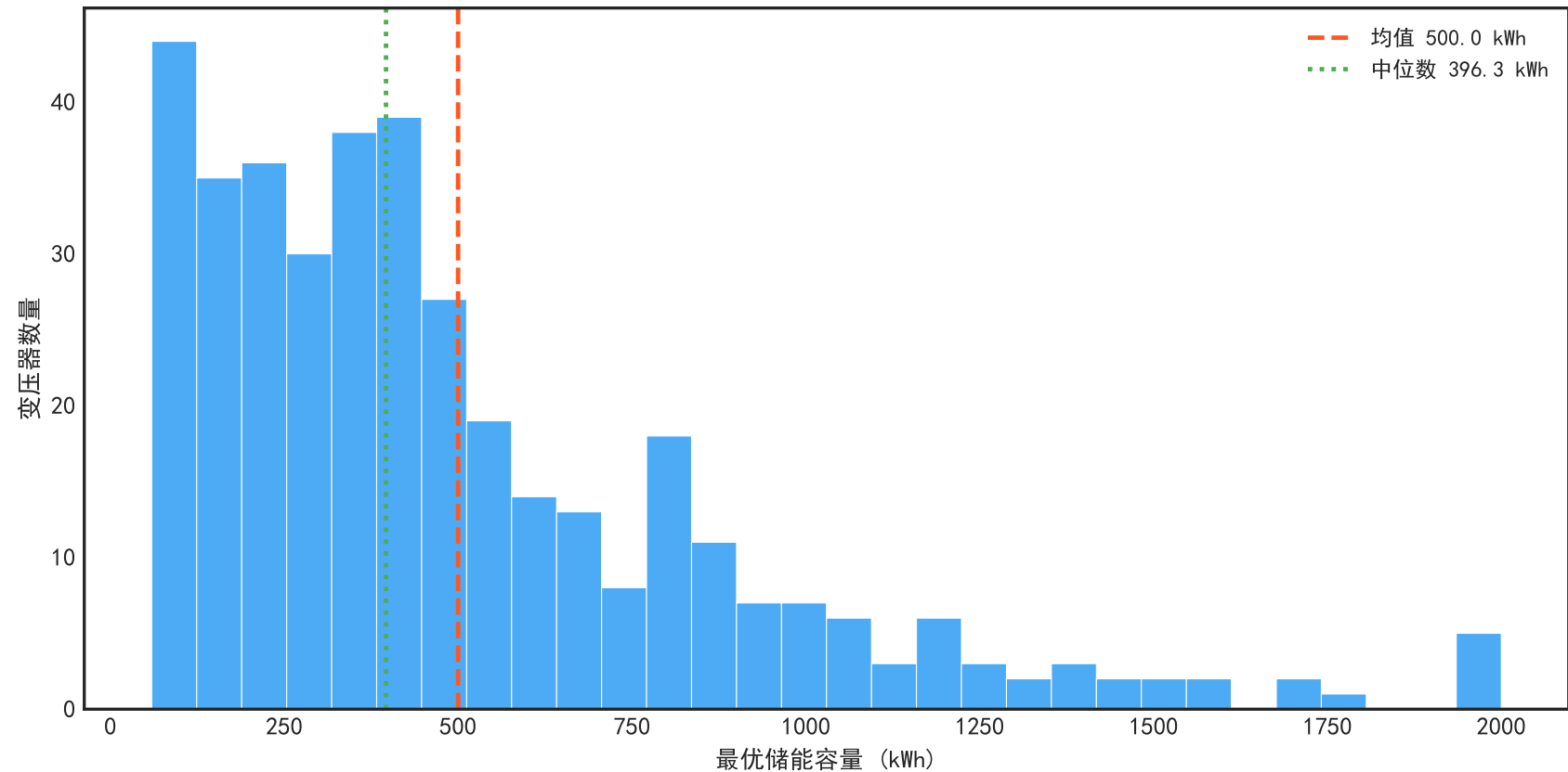
最优储能容量分布 (n=383) unit_cost=1500.0 元/kWh, lifetime=10.0 年
