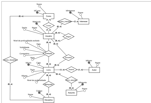
Figure: Modelo Entidade-Relacionamento do sistema UnBooks
