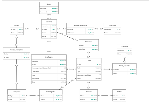
Figure: Diagrama Entidade-Relacionamento do sistema UnBooks
