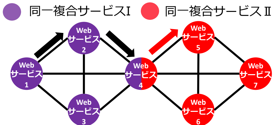
ランダムウォーク
