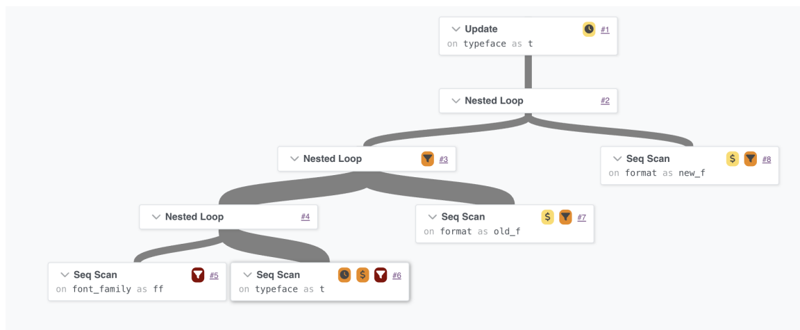
Рис. 25: План выполнения запроса 9
