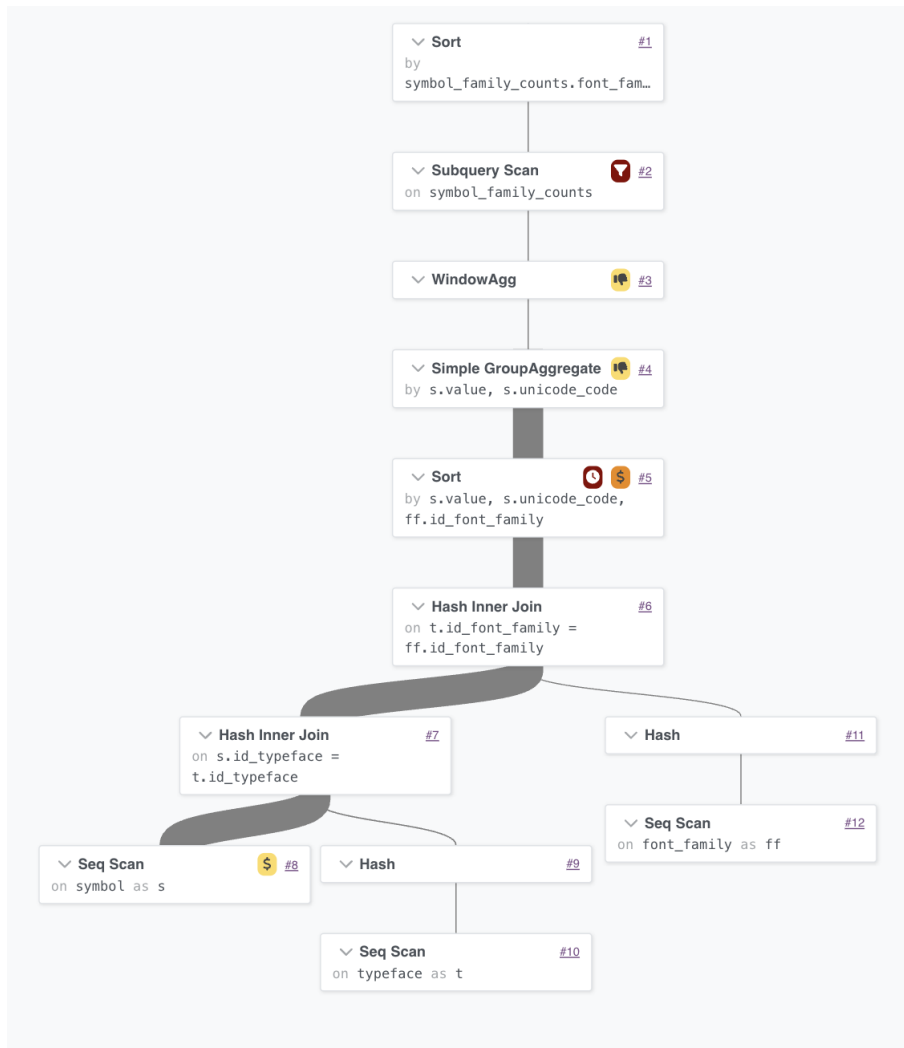
Рис. 17: План выполнения запроса 5
