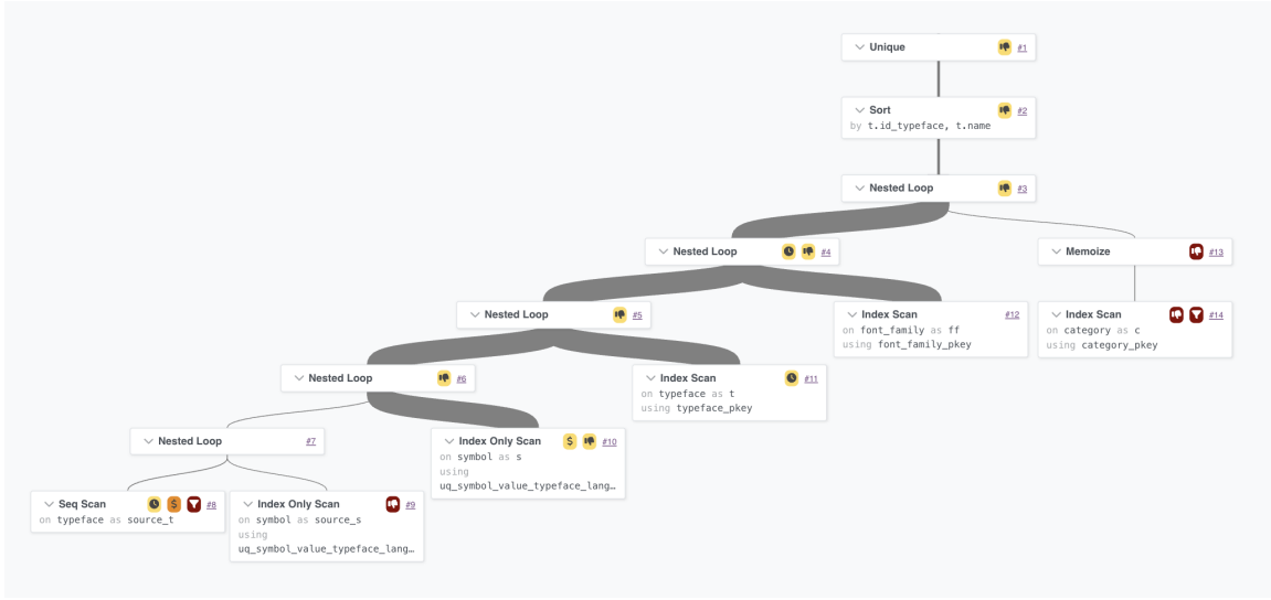
Рис. 8: План выполнения запроса 1
