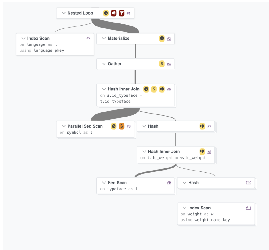
Рис. 19: План выполнения запроса 6
