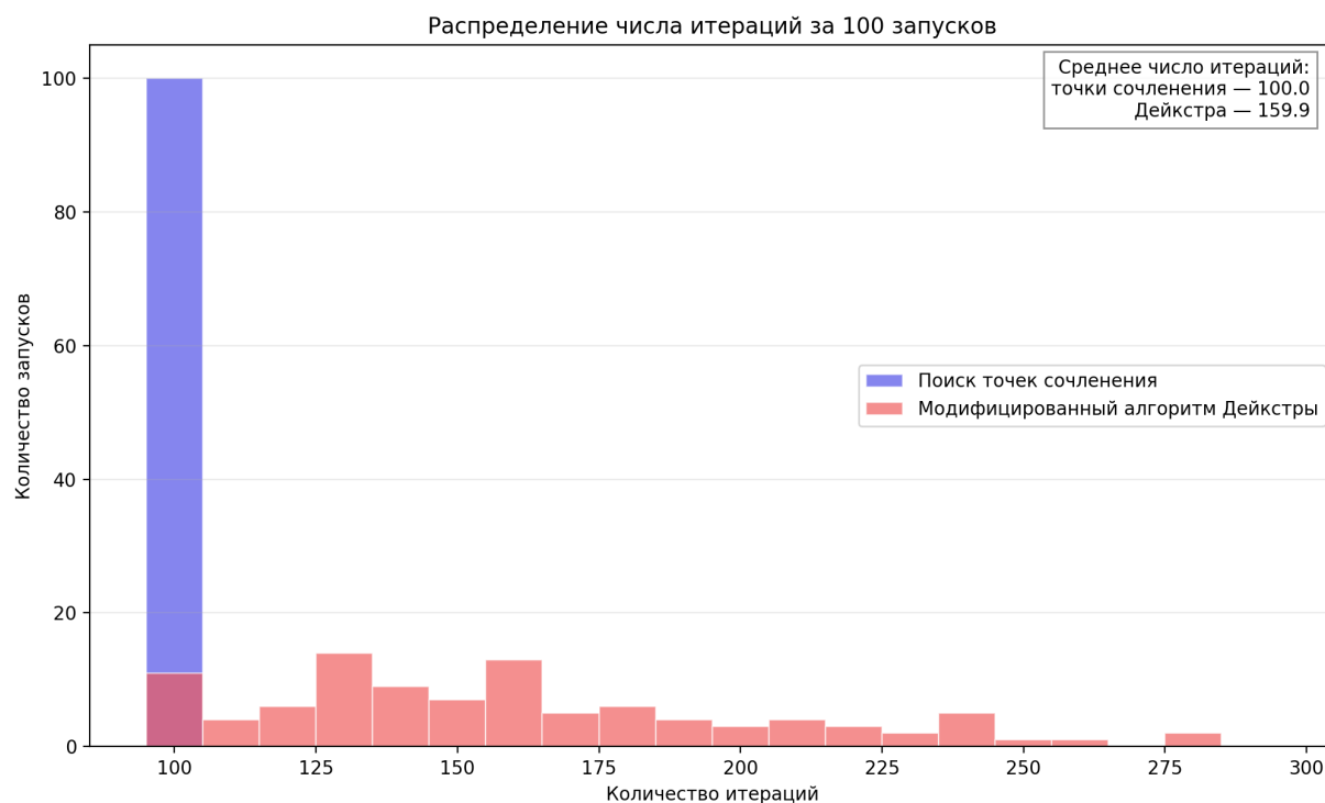
Рис. 27: Распределение количества итераций за 100 запусков
