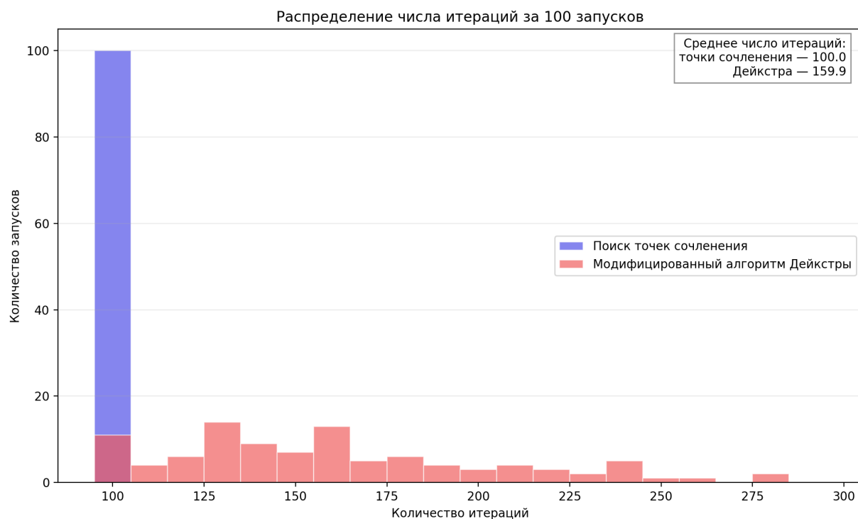
Рис. 26: Распределение количества итераций за 100 запусков
