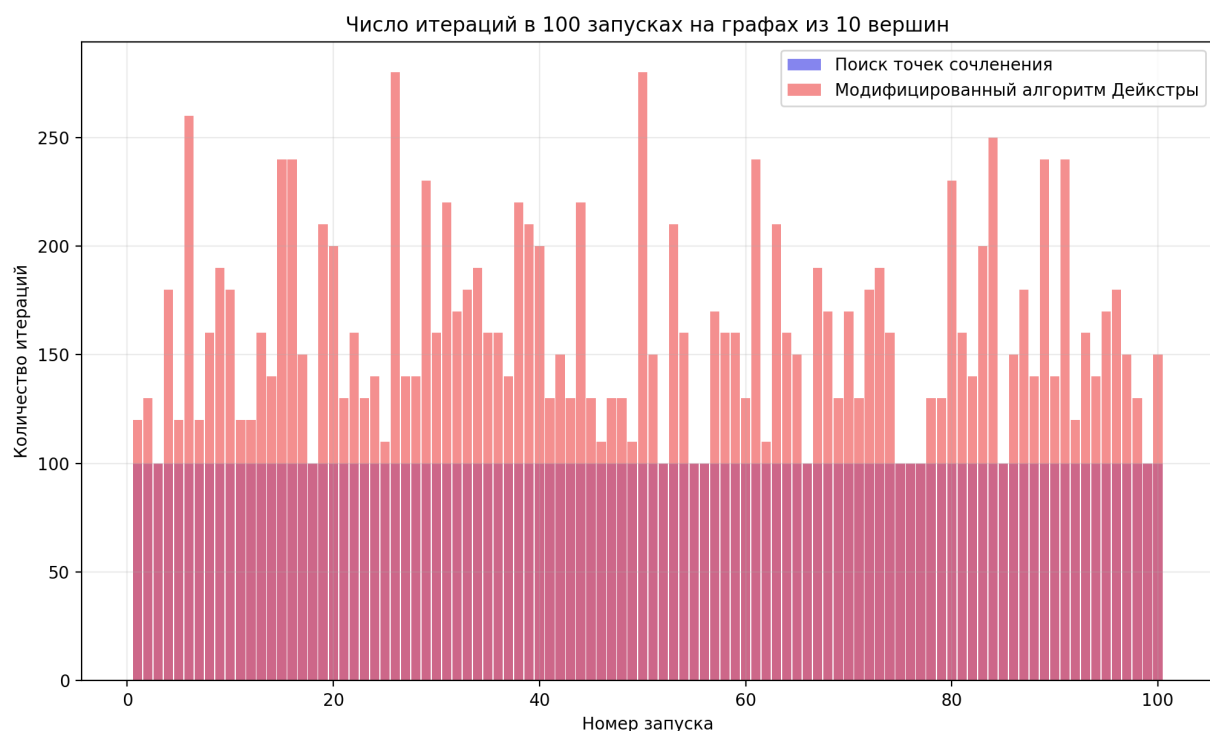
Рис. 25: Количество итераций в каждом запуске
