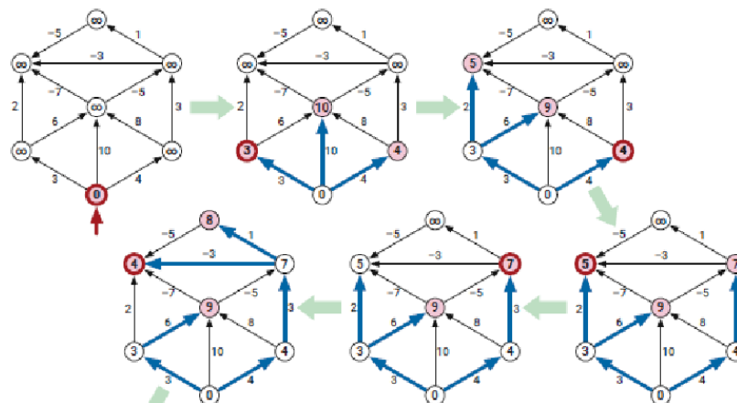
Рис. 7: Последовательное изменение весов при работе алгоритма, часть 1
